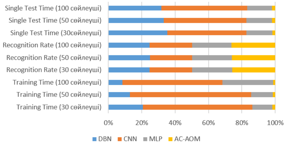
6-сурет. Төрт түрлі тану әдісі үшін тану жылдамдығы
