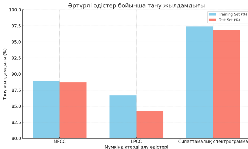
5-сурет. Әртүрлі әдістер бойынша тану жылдамдығы
